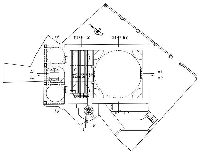
γενική κάτοψη κτιρίου
